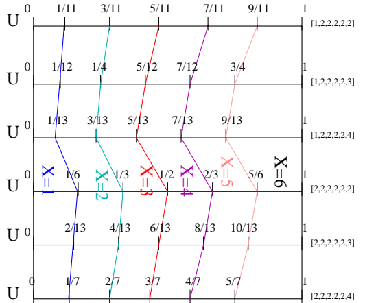
FIG. 2 – Simulation de valeur pour un dé biaisé
